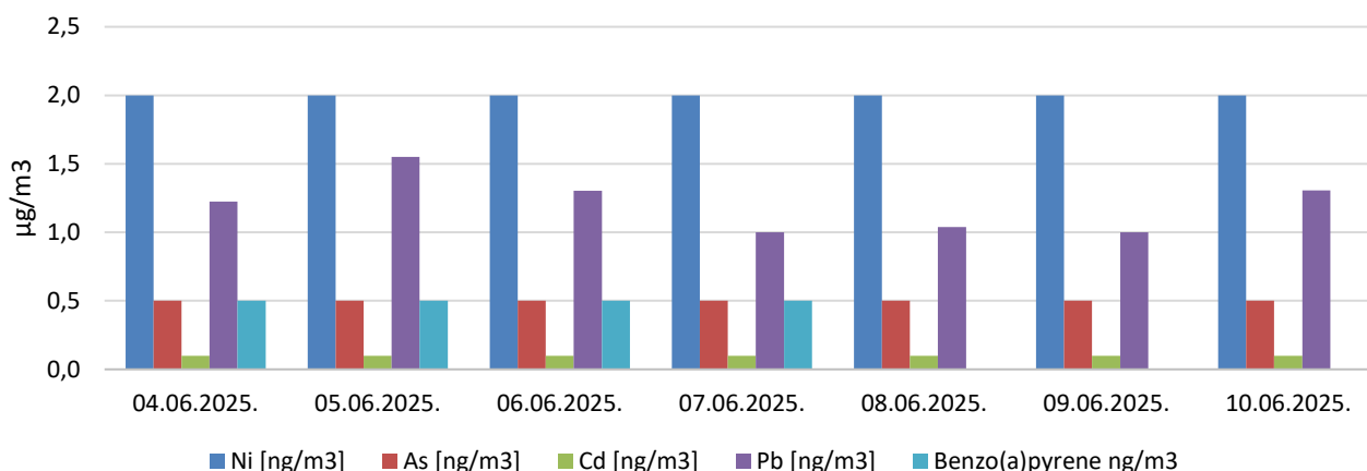
MM1 Метали у суспендованим честицама PM10 у периоду 4.6.-10.6.2025.
