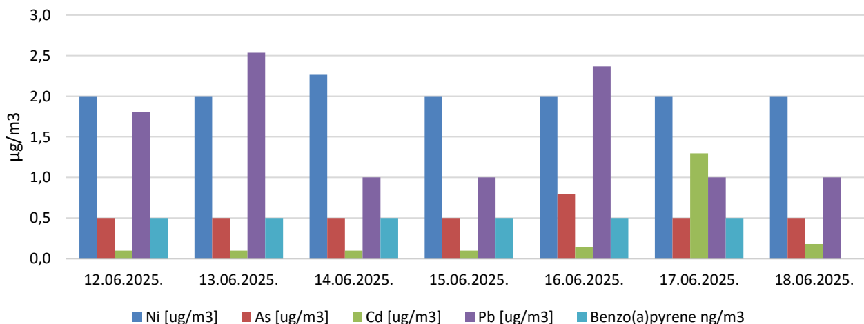
MM2 Метали у суспендованим честицама PM10 у периоду 12.6.-18.6.2025.
